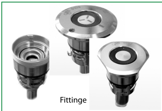
Korb-, Flach-, Dreikant- und Kombizapfköpfe
